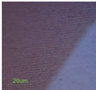
Variable pitched grooves (Logo) 可変ピッチ溝パターン (ロゴ)
